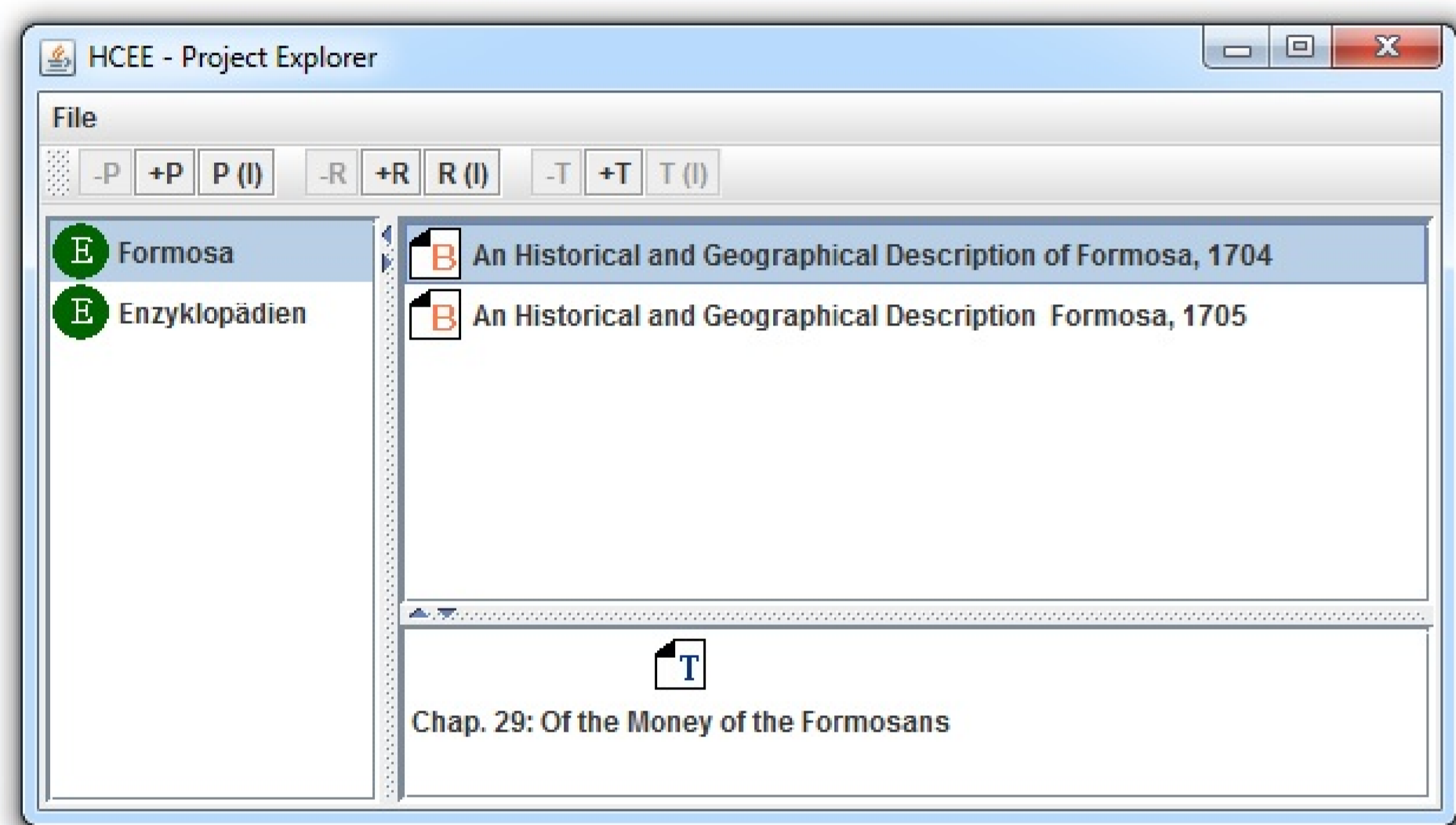
Screenshot HCEE – Projektwahl
