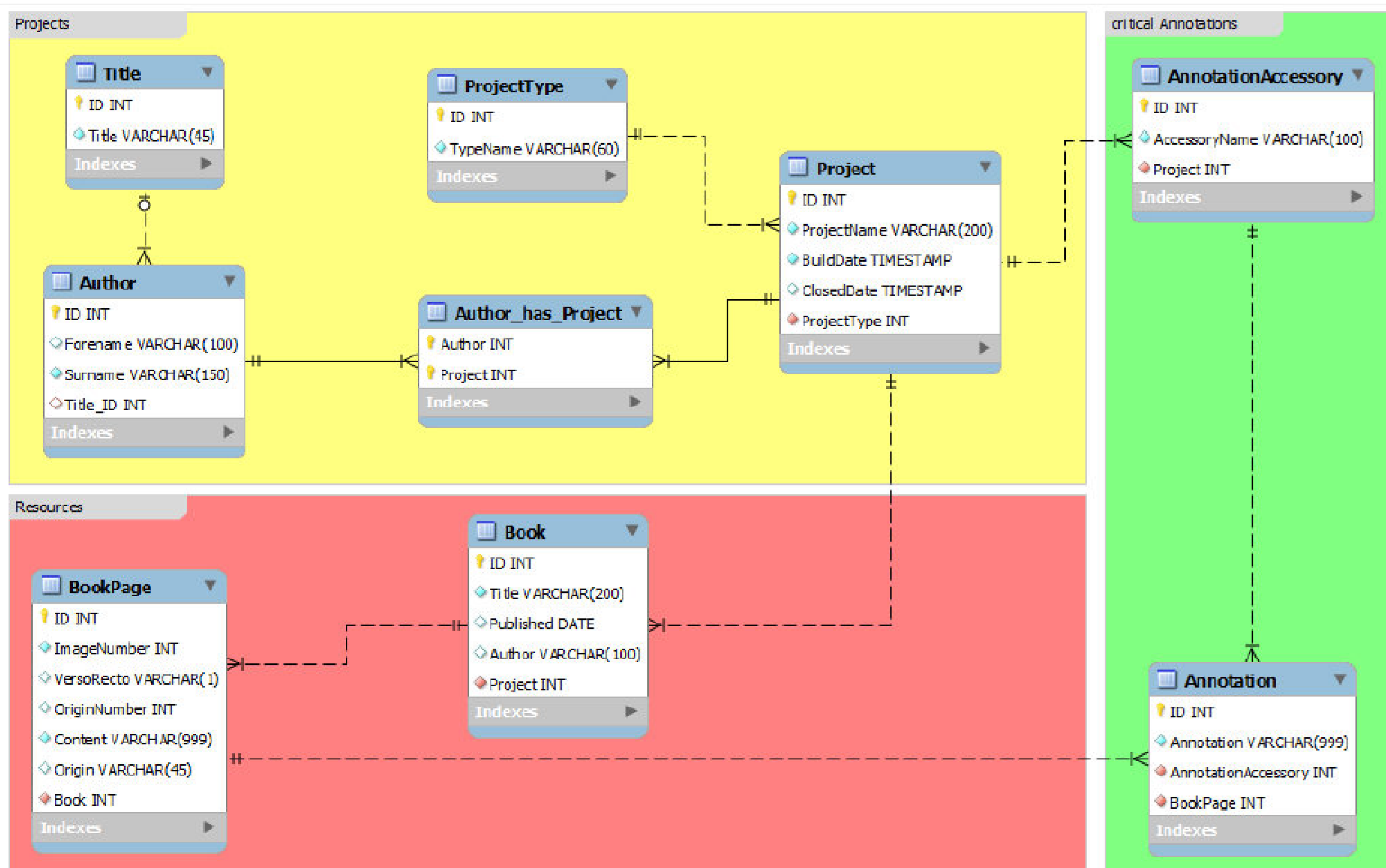
Datenbank-Schema HCEE und HCEV
